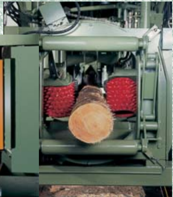
Einzugsaggregat
